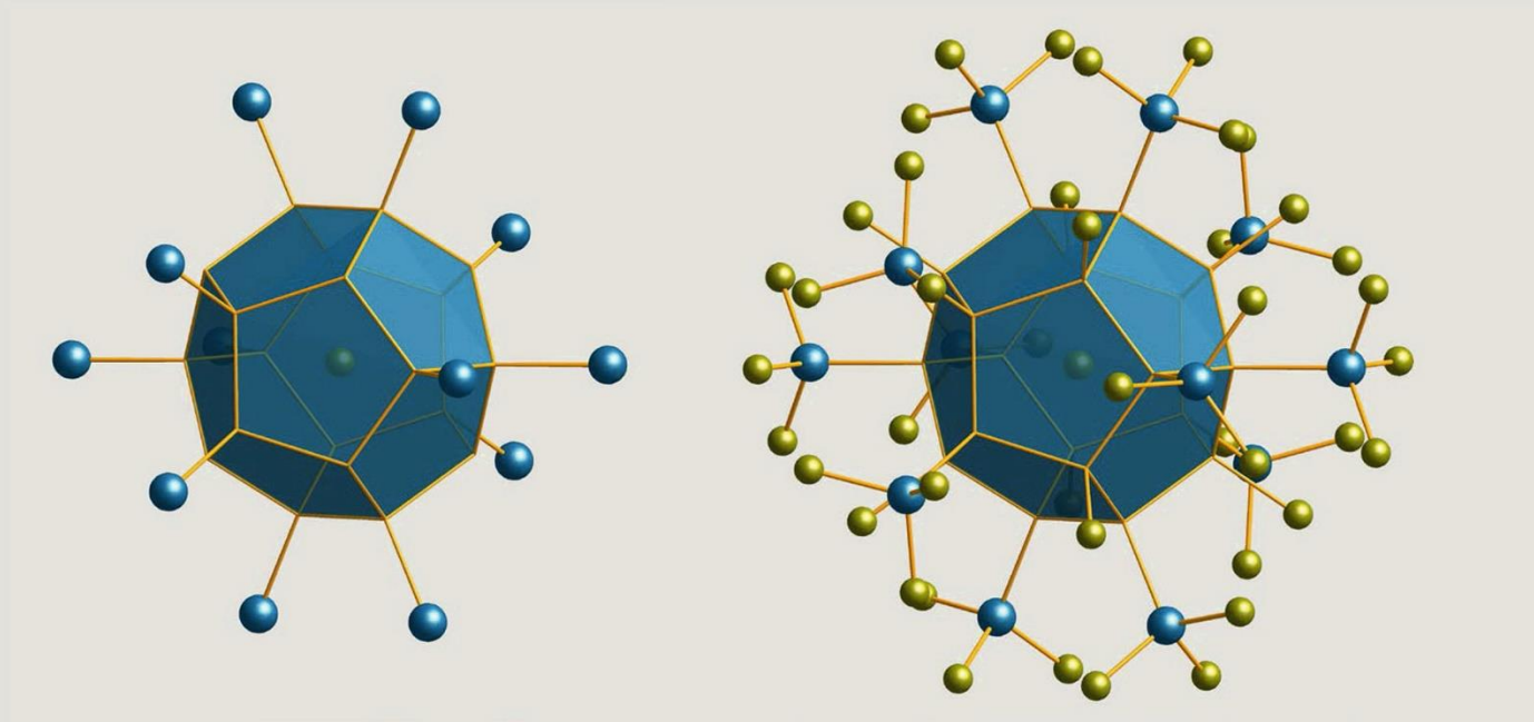
2015: Erstes Silafulleran
